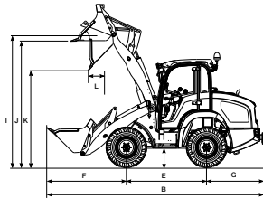
Radlader mit Standardschaufel und Standardbereifung (Seitenansicht)
