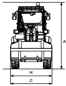
Radlader mit Standardschaufel und Standardbereifung (Frontansicht)
